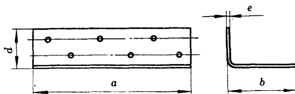
图 1 底座用起吊护铁的结构型式(内装物在 6 000 kg 以下)
